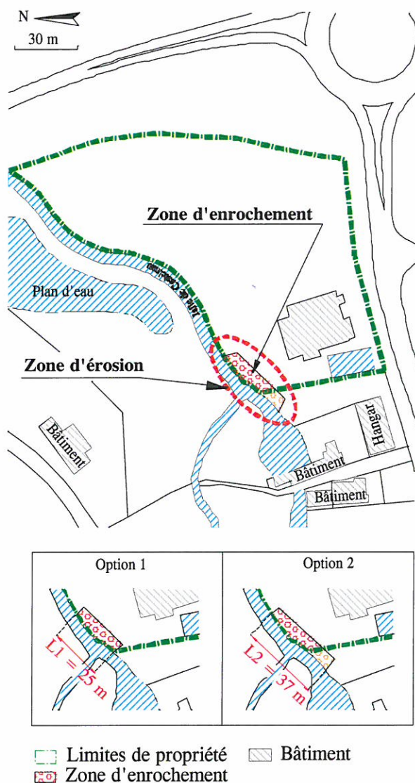
Figure n°27 : Plan de la zone d'enrochement. (04.010.A.AF(R.01.1).27.1)
